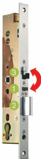
EL 520 (Axes à 50, 55, 60 et 65 mm) EL 420 (Axes à 30, 35, 40 et 45 mm)
